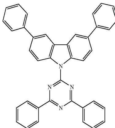
[CT]
