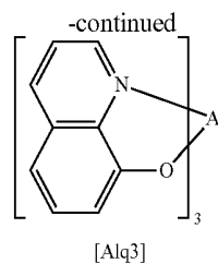
[Alq 3 ]
