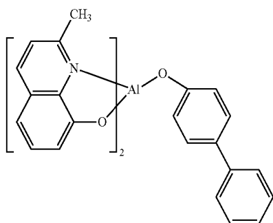
[BALq]
